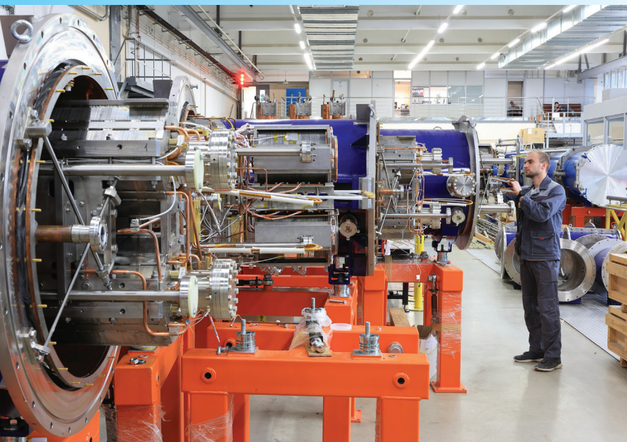
Фабрика сверхпроводящих магнитов
