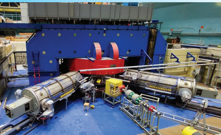
Модернизированный ускоритель У-400М
