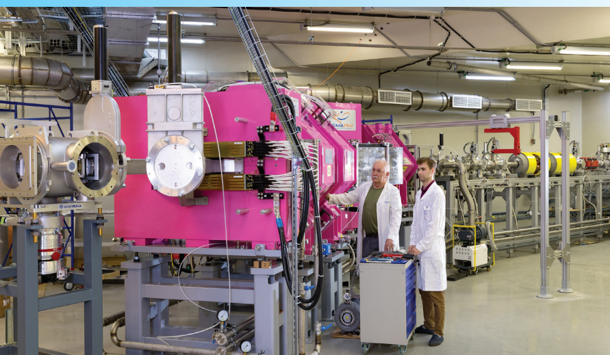
Газонаполненный сепаратор GRAND, Фабрика СТЭ
