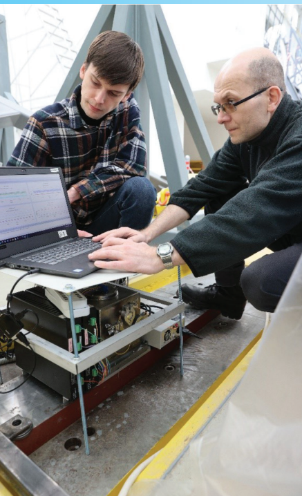
Установка малогабаритного лазерного инклинометра в зале MPD NICA
