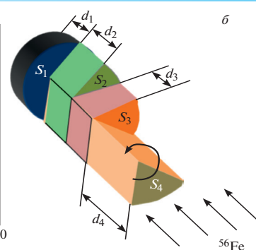
а) Сравнение расчетных зарядовых распределений частиц во внутреннем радиационном поле космического корабля в минимуме и максимуме солнечной активности и в поле за симулятором; б) схематический вид конвертора симулятора
