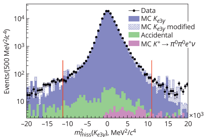
Распределение квадрата недостающей массы комбинаций зарегистрированных частиц \pi^0 e^+ \nu для отобранных экспериментальных событий (точки), а также для ожидаемого сигнала и фона (гистограммы)
