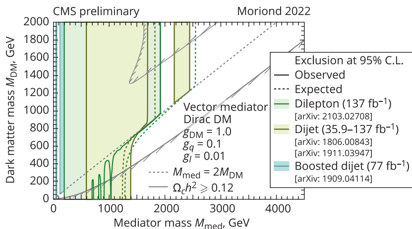
Пределы (95% C.L.) на массы частицы темной материи M_{DM} и векторной частицы-переносчика взаимодействия с темным сектором M_{med} (закрашенная область). Результаты основаны на данных, полученных в RUN-2 в объединенном канале рождения пары струй и пары лептонов
