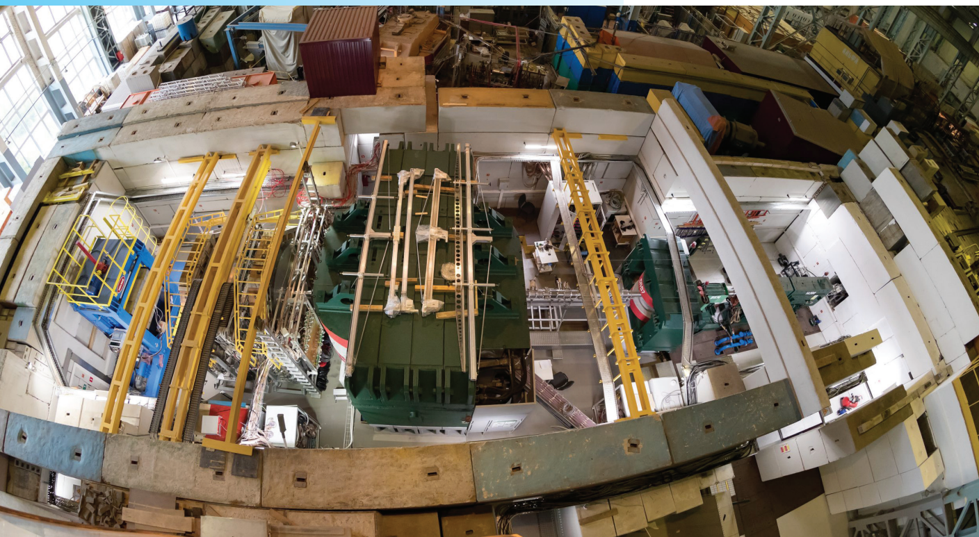
Общий вид экспериментальной зоны BM@N (осень 2022 г.)
