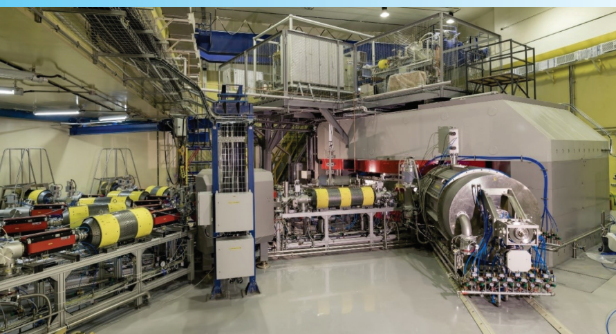
Циклотрон ДЦ-280, Фабрика СТЭ
