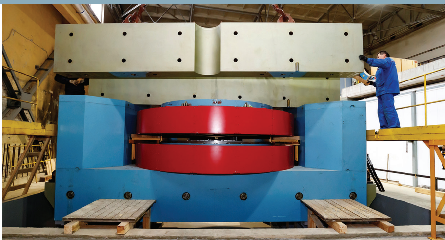
Монтаж циклотрона ДЦ-140
