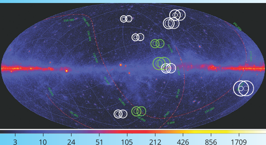
Положение первых 10 кандидатов на астрофизические нейтринные события в Baikal-GVD на небесной карте с источниками FERMI-LAT в галактической системе координат. Внутренняя и внешняя окружности вокруг событий соответствуют вероятности регистрации 50 и 90 %
