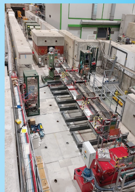
ЦЕРН (Женева). Установка NA64 на мюонном (слева) и электронном (справа) каналах ускорителя SPS
