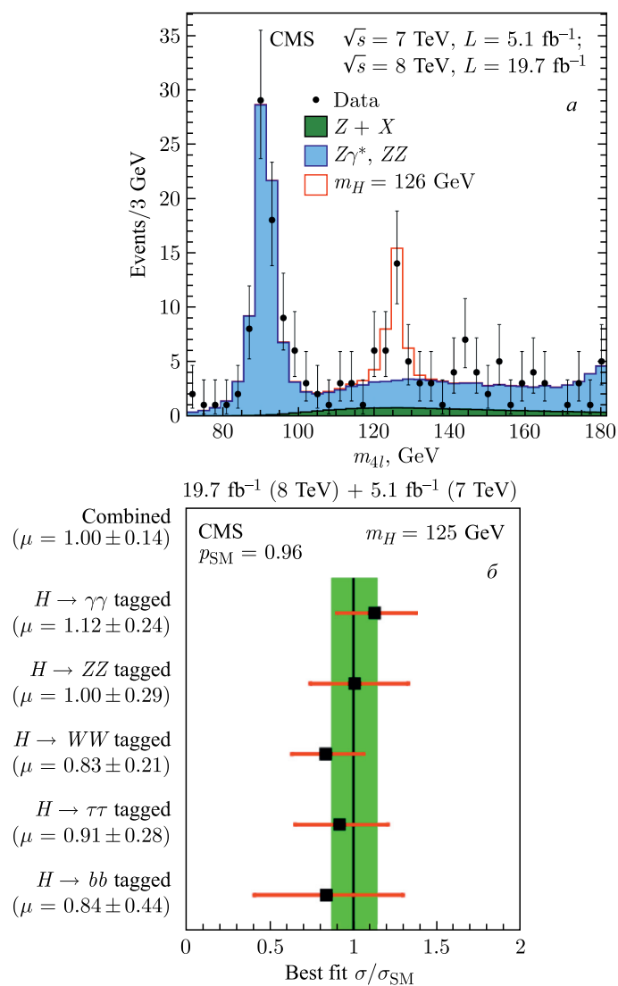
Рис. 1. a ) Распределение по инвариантной массе четырех лептонов. б ) Интенсивность сигнала бозона Хигса
