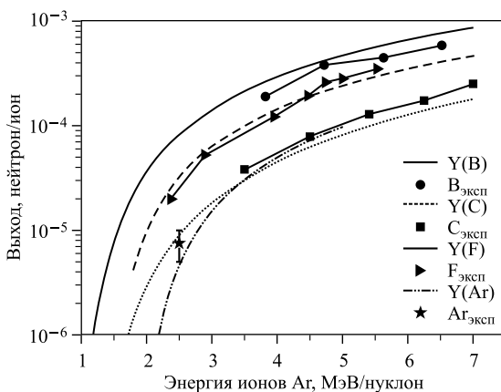
Рис. 2. Выходы нейтронов при бомбардировке мишени из Al пучками ионов бора, углерода, фтора и аргона в зависимости от энергии. Y(\text{B}) , Y(\text{C}) , Y(\text{F}) и Y(\text{Ar}) — выходы нейтронов при бомбардировке мишени из алюминия ионами бора, углерода, фтора и аргона, рассчитанные по программе LISE ++ , точки — экспериментальные значения из [1] и значение для аргона, полученное на ускорителе ДЦ-110
