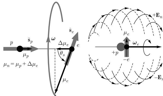
Рис. 4. Свойства нейтрона: слева — прецессия электрона (чтобы изображение прецессии электрона было наглядным, угол \theta_s изображен гораздо меньшим, чем он может быть на самом деле — близким к 90^\circ , таким он изображен справа); справа — электрическое поле нейтрона, созданное прецессией входящего в его состав электрона (воспроизведены рисунки из книги [2] со с. 137 и 138)
