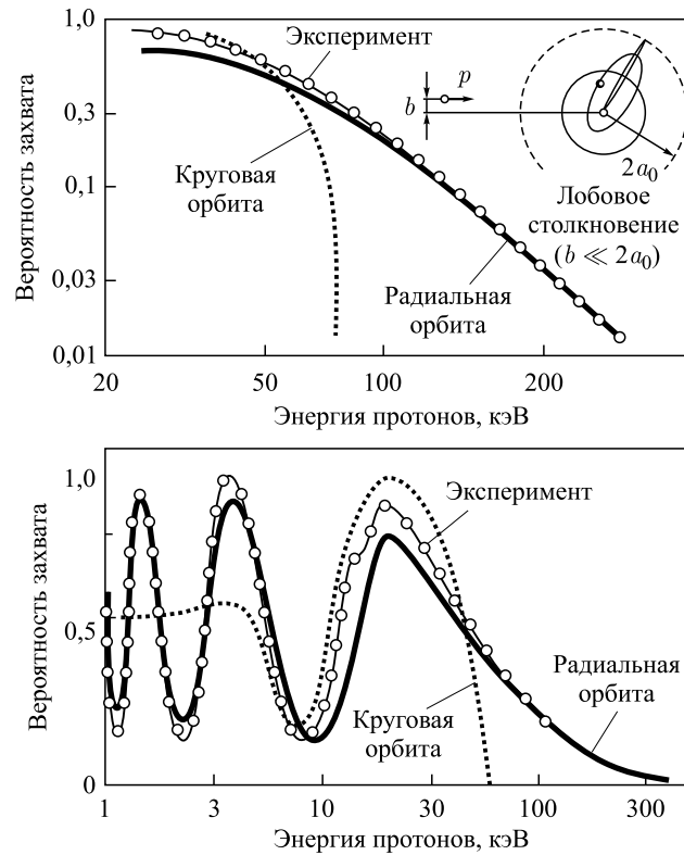
Рис. 1. Захват электрона в лобовом столкновении протонов с атомами водорода: сравнение результатов теоретических вычислений вероятности захвата для разных типов кинетики (радиальной и круговой) атомных электронов с данными эксперимента (воспроизведен рис. 1 из работы [4])
