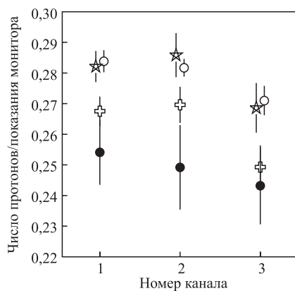
Рис. 10. Отношения чисел протонов к показаниям монитора, усредненные по всем экспозициям, для мишеней T1 разной толщины: черные кружки — 137 \text{ г/см}^2 , звездочки — 83 \text{ г/см}^2 , крестики — 54 \text{ г/см}^2 , светлые кружки — 0 \text{ г/см}^2
