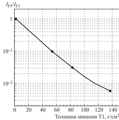
Рис. 2. Отношения интенсивностей в фокусах F5 и F3 для мишеней T1 разной толщины, зарегистрированные ионизационными камерами
