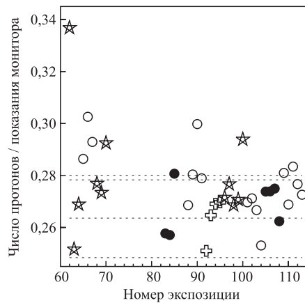
Рис. 4. Отношения чисел протонов к показаниям монитора ( M1b + M2b ) в фокусе F5 для мишеней T1 разной толщины: черные кружки — 137 г/см 2 , звездочки — 83 г/см 2 , крестики — 54 г/см 2 , светлые кружки — 0 г/см 2
