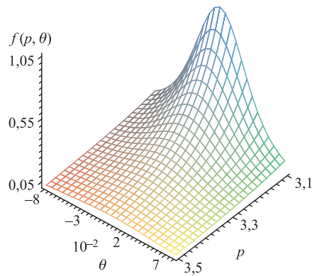
Рис. 6. Инвариантное дифференциальное сечение f(p, \theta) = (E/p^2)d^2\sigma/d\Omega dp (в единицах мб/ср \cdot ГэВ 2 /с 3 ) испускания протонов в реакции стриппинга дейтронов с импульсом 5 ГэВ/с в зависимости от импульса (в ГэВ/с) и угла вылета \theta (в рад) протона в лабораторной системе
