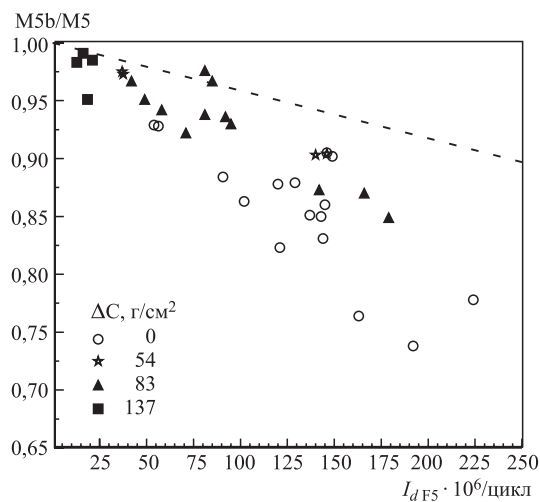
Рис. 9. Зависимость отношения числа заблокированных отсчетов монитора M5 к числу неблокированных от интенсивности пучка в сбросе в фокусе F5 . Пунктиром показана расчетная зависимость в случае блокировки аппаратуры на время считывания данных при отсутствии модуляции растяжки
