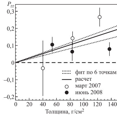
Рис. 11. Тензорная поляризация дейтронов в зависимости от толщины углеродной мишени Т1. Светлые точки — результаты работы [9], черные точки — результаты настоящей работы. Штриховые линии ограничивают коридор ошибок. Сплошная кривая — результат вычисления P_{ZZ} в рамках модели многократного рассеяния [17]
