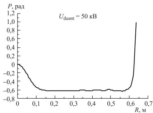
Рис. 3. Фазовое движение
