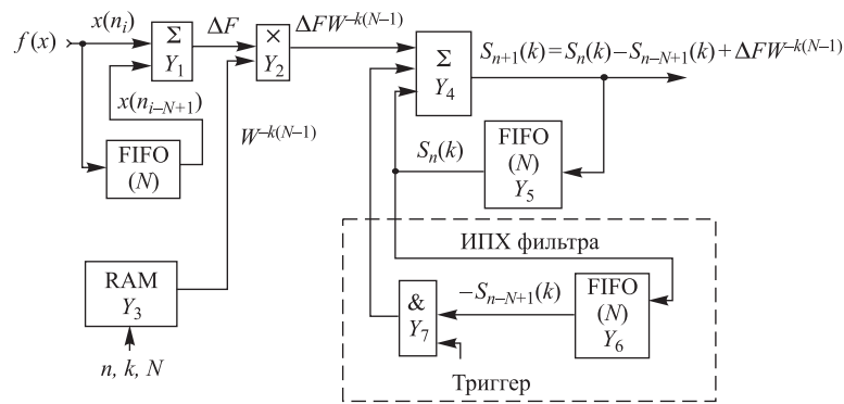
Рис. 2. Функциональная схема реализации алгоритма активной фильтрации на базе РПФ
