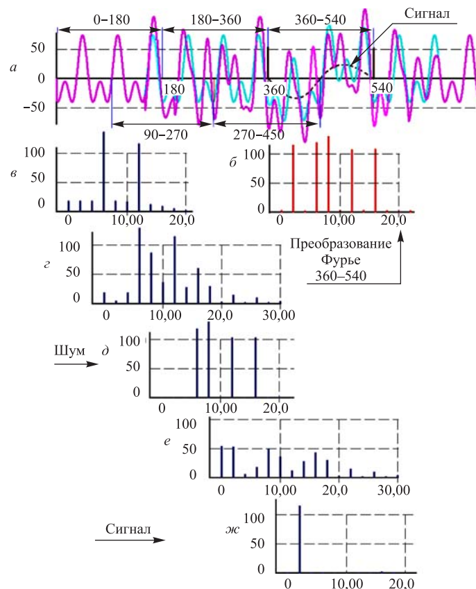
Рис. 3. Временные диаграммы работы алгоритма активной фильтрации: а) временная диаграмма регистрируемого сигнала, содержащего полезный (гармонический) сигнал и шумовую компоненту, б) спектральное преобразование Фурье регистрируемого сигнала, в-е) спектральные оценки РПФ, вычисленные в различные моменты времени, ж) спектр полезного сигнала, «очищенный» от шума
