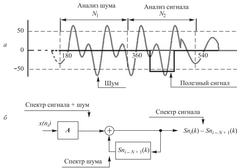
Рис. 1. Реализация алгоритма активной фильтрации: а) временная диаграмма работы алгоритма, б) функциональная блок-схема алгоритма фильтрации
