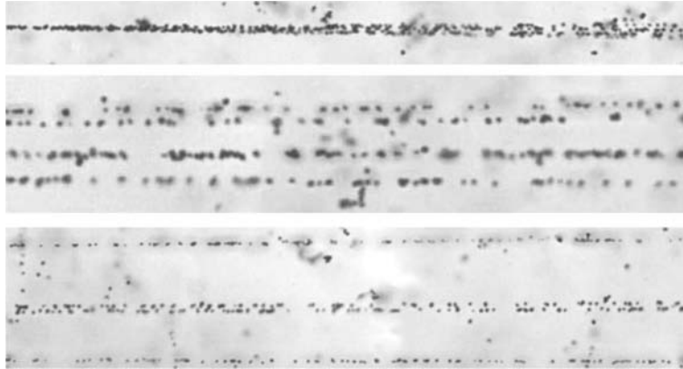
Рис. 8. Фрагментация релятивистского ядра \text{Ne} \rightarrow 5\text{He} с импульсом 4,5 \text{ А ГэВ/с} в периферическом взаимодействии на ядре эмульсии; на верхней фотографии видна вершина взаимодействия и струя фрагментов в очень узком угловом конусе; среднее фото: смещение от вершины взаимодействия по направлению движения фрагментов, становятся различимыми три фрагмента \text{He} и очень узкая пара треков; нижнее фото: дальнейшее смещение вдоль струи фрагментов с целью разделения узкой пары \text{He} фрагментов, являющихся продуктами промежуточного нестабильного ядра {}^8\text{Be}
