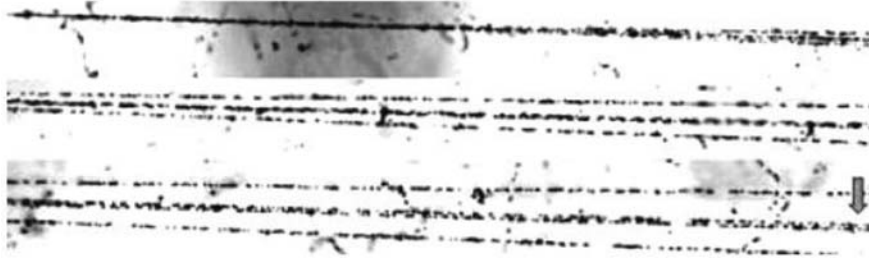
Рис. 7. Фрагментация релятивистского ядра ^{16}\text{O} \rightarrow 4\text{He} с импульсом 4,5 А ГэВ/с в периферическом взаимодействии на ядре эмульсии. На верхней фотографии видна вершина взаимодействия и струя фрагментов в очень узком угловом конусе; среднее фото: смещение от вершины взаимодействия по направлению движения фрагментов, становятся различимыми два фрагмента He и очень узкая пара треков; нижнее фото: дальнейшее смещение вдоль струи фрагментов с целью разделения узкой пары фрагментов He, являющихся продуктами промежуточного нестабильного ядра ^8\text{Be}
