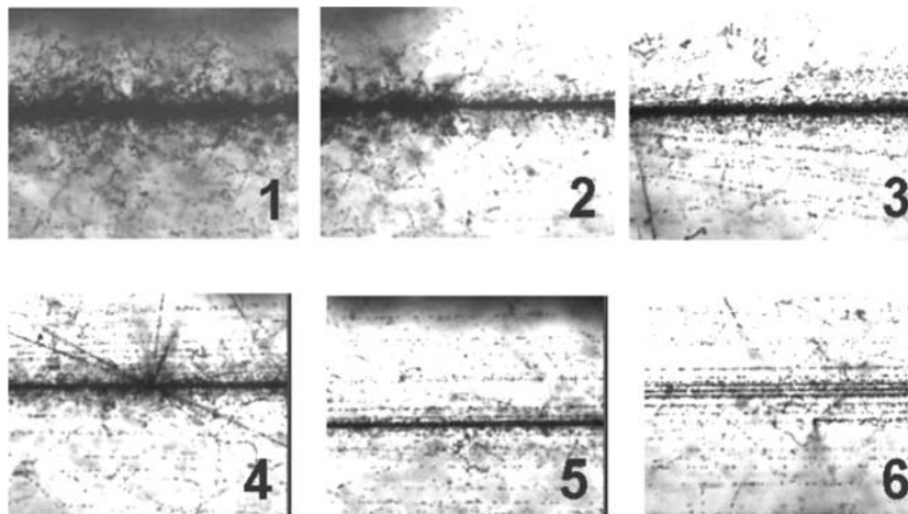
Рис. 9. Последовательные фотокадры когерентной диссоциации ядра \text{Pb} при 160 \text{ А ГэВ} : первичный след (1), вершина диссоциации (2), расхождение следов (3–6); на 4-м кадре видна первая вторичная вершина; 6-й кадр соответствует удалению от вершины около 3 \text{ см}
