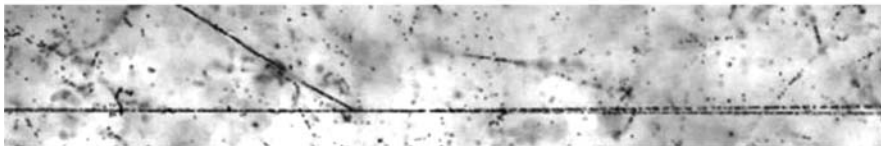
Звезда с тяжелым осколком ( b -частицей)
