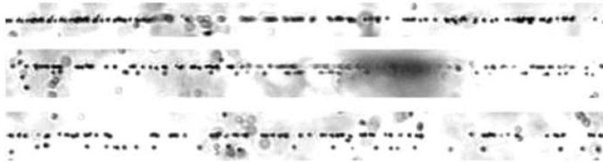
Рис. 10. Фрагментация релятивистского ядра {}^6\text{Li} на одно- и двухзарядный фрагмент в эмульсии; на верхней фотографии видна вершина взаимодействия и узкая струя из двух фрагментов; при смещении вдоль струи фрагментов (нижние фотографии) отчетливо разделяются один однозарядный и один двухзарядный фрагменты
