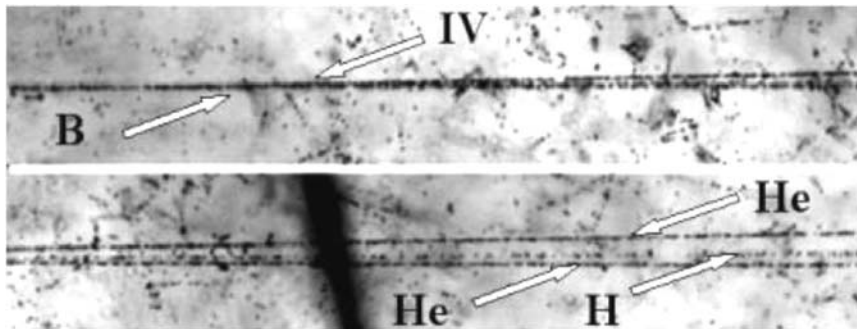
Рис. 21. Диссоциация ядра {}^8\text{B} \rightarrow 2\text{He} + \text{H} с энергией 1,2 А ГэВ в периферическом взаимодействии на ядре эмульсии. На верхней фотографии видна вершина взаимодействия и струя фрагментов в узком угловом конусе. При смещении по направлению струи фрагментов (нижняя фотография) можно различить 2 фрагмента He и фрагмент H (трек в середине)
