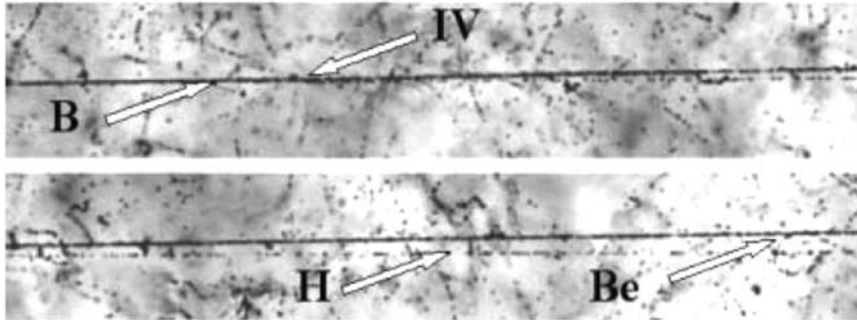
Рис. 20. Диссоциация ядра {}^8\text{B} \rightarrow {}^7\text{Be} + p с энергией 1,2 А ГэВ в периферическом взаимодействии на ядре эмульсии. На верхней фотографии указана вершина взаимодействия IV. При смещении по направлению струи фрагментов (нижняя фотография) можно различить фрагмент Be и фрагмент H
