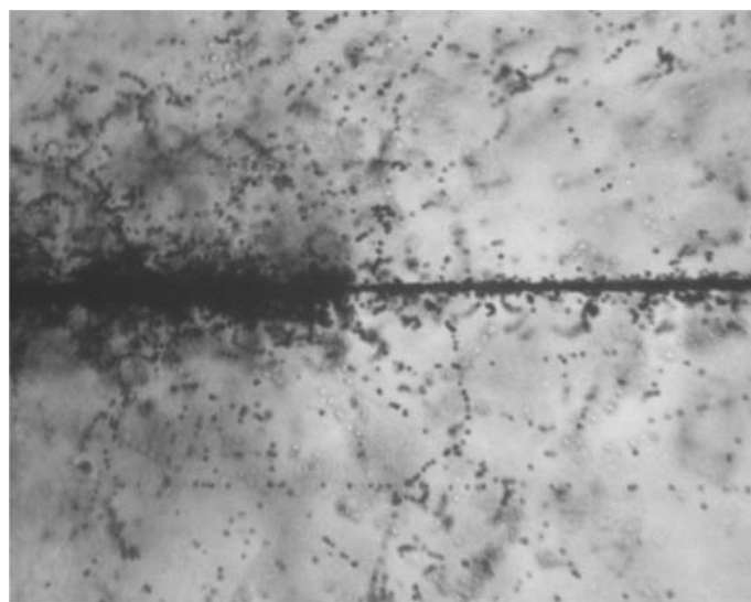
Рис. 5. Периферическое соударение ядра Au с энергией 10,7 А ГэВ с ядром из состава ядерной эмульсии
