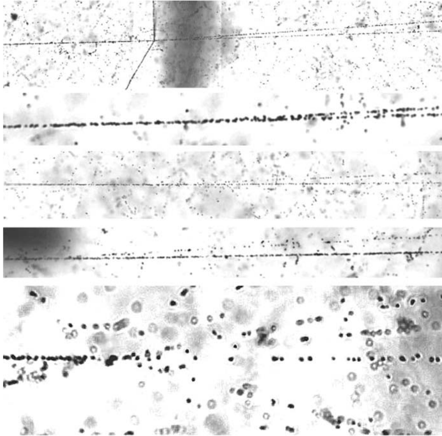
Рис. 17. Примеры событий периферической диссоциации ядра {}^7\text{Be} в эмульсии; на верхней фотографии — расщепление на два фрагмента He с образованием двух осколков ядра мишени; ниже — «белые звезды» с расщеплением на 2\text{He} , \text{He} + 2\text{H} , \text{Li} + \text{H} и 4\text{H}
