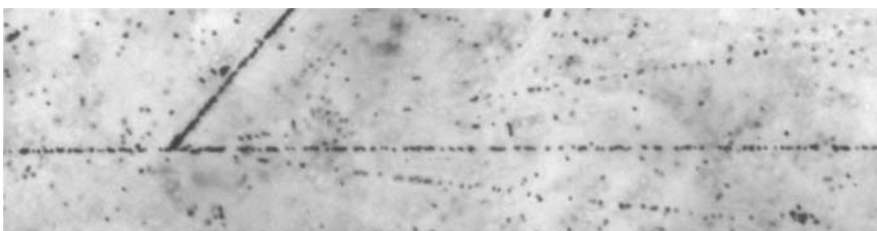
Рис. 12. Событие фрагментации {}^6\text{He} \rightarrow {}^4\text{He} : входящая слева частица с зарядом Z_{\text{пр}} = 2 создала вершину взаимодействия с фрагментом мишени, парой мезонов и почти не отклоняющийся релятивистский фрагмент Z_{\text{фр}} = 2
