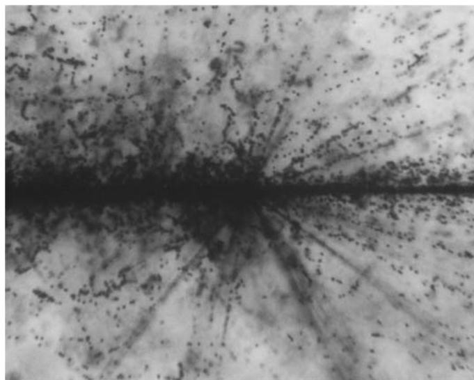
Рис. 4. Центральное соударение ядра Au с энергией 10,7 А ГэВ с ядром из состава ядерной эмульсии
