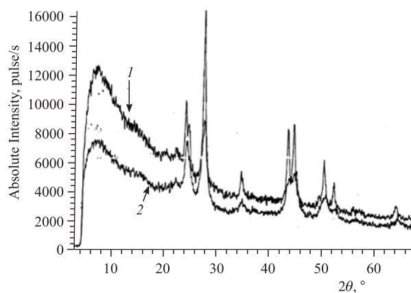
Рис. 1. Дифрактограммы образцов, полученных методом соосаждения: 1 — \text{LaF}_3 ; 2 — \text{La-F-Hf}
