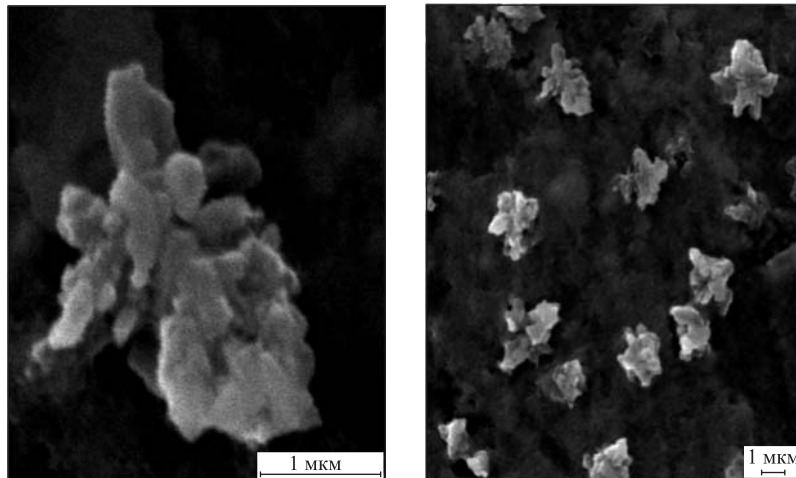
Рис. 4. Электронно-микроскопические снимки продуктов частичной кристаллизации, полученных при соосаждении ионов Hf с \text{LaF}_3 из фторидных водных растворов в масштабе 1 мкм
