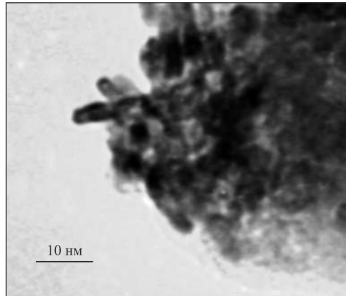
Рис. 2. Электронно-микроскопический снимок (ПЭМ) агрегатов первичных аморфных частиц, полученных при сосаждении ионов Hf с \text{LaF}_3 из фторидных водных растворов
