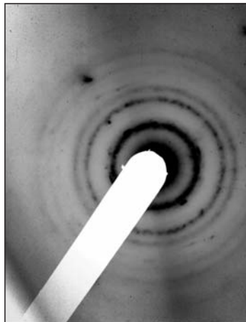
Рис. 3. Электронограмма частицы с зародышами кристаллов, полученной при сосаждении ионов Hf с \text{LaF}_3 из фторидных водных растворов
