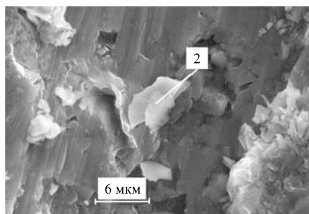
Рис. 5. СЭМ-изображение поверхности Al. РМЗА был сделан в выделенной точке 2
