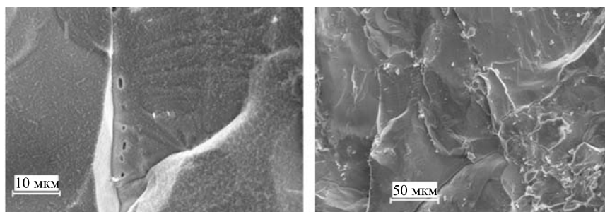
Рис. 4. СЭМ-изображения исходного слитка YMn 2 с различным увеличением. РМЗА был сделан для всей площади поверхности образца
