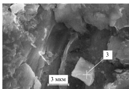
Рис. 6. СЭМ-изображение поверхности Al. РМЗА был сделан в выделенной точке 3
