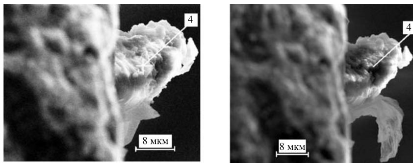
Рис. 8. Два СЭМ-изображения поверхности Al с застывшим выбросом, который в процессе экспозиции для ХСРИ изменил форму (переплавился)
