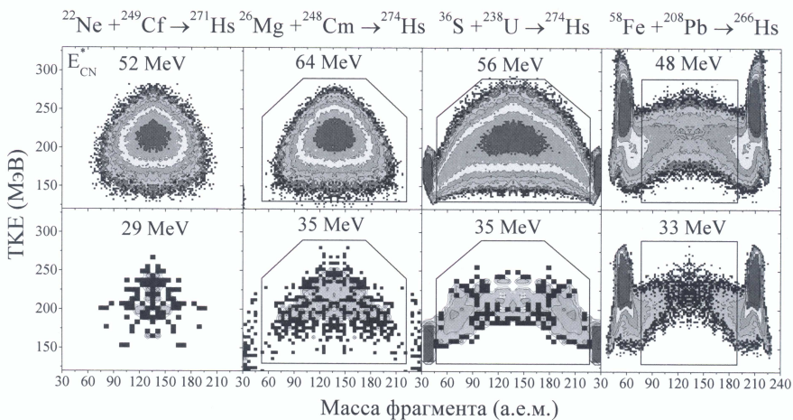
Рисунок 1. Двумерные распределения выходов фрагментов реакций в зависимости от их массы и полной кинетической энергии ( M , ТКЕ).
