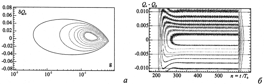
Рис. 3. Карты: (а) изолиний \alpha(g, \delta Q_0) = \alpha_l [4] и (б) изоамплитуд a_e(n, Q_c - Q_\beta) = a_l [5]
