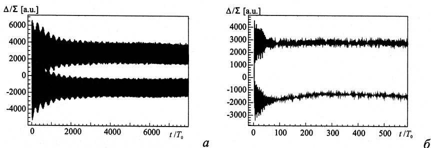
Рис. 6. Подавление горизонтальных ошибок при инжекции (beam 1) при выключенной (а) и включенной (б) СП; сигналы с датчиков Q7 (верхний луч) и Q9 (нижний луч) [25]
