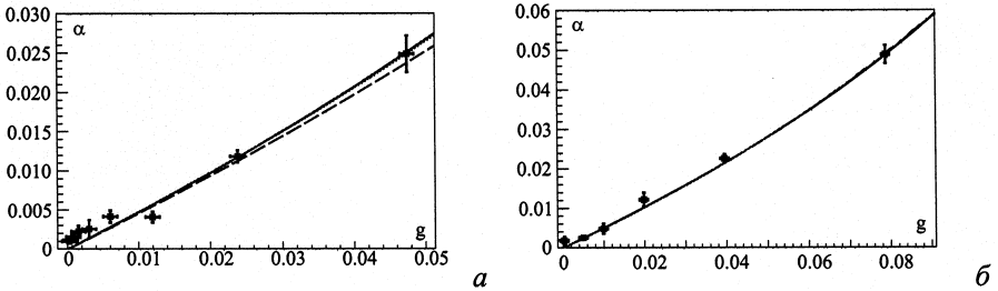
Рис. 2. Расчетные декременты затухания и результаты измерений горизонтальных (а) и вертикальных (б) когерентных поперечных колебаний пучка протонов с энергией 3.5 ТэВ в ЛНС [5, 15]
