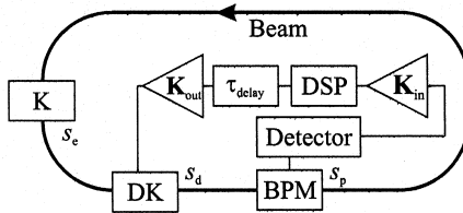
Рис. 1. Структурная схема цифровой системы подавления когерентных колебаний пучка [L2]
