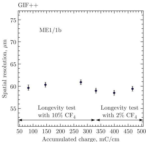
Рис. 6. Пространственное разрешение ME1/1b, измеренное в пучке мюонов на установке GIF++ в период облучения камеры с рабочей газовой смесью, содержащей 10% \text{CF}_4 (данные отложены до величины накопленного заряда 332 МКл/см включительно), и в период облучения камеры с газовой смесью, содержащей 2% \text{CF}_4 (выше 332 МКл/см)
