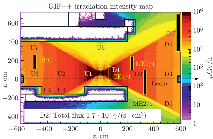
Рис. 3. Карта интенсивности радиационного поля источника ^{137}\text{Cs} установки GIF++ [11]. Указаны позиции детекторов, расположенных в зоне облучения
