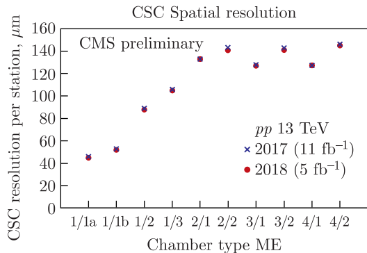
Рис. 2. Пространственное разрешение мюонных станций ME в период набора данных CMS в p-p -столкновениях в 2017–2018 гг.
